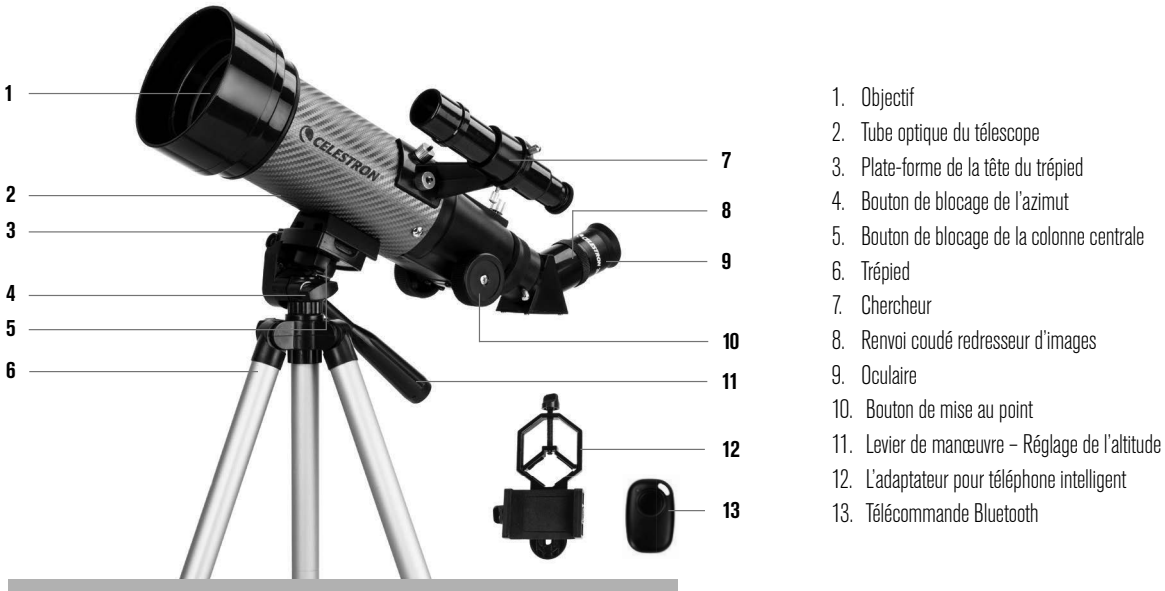
Fig. 1 Longue vue de voyage 70DX (Similaire au Travel Scope 60DX)
