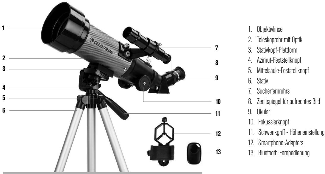
Abb. 1 Travel Scope 70DX (Travel Scope 60DX ähnlich)
