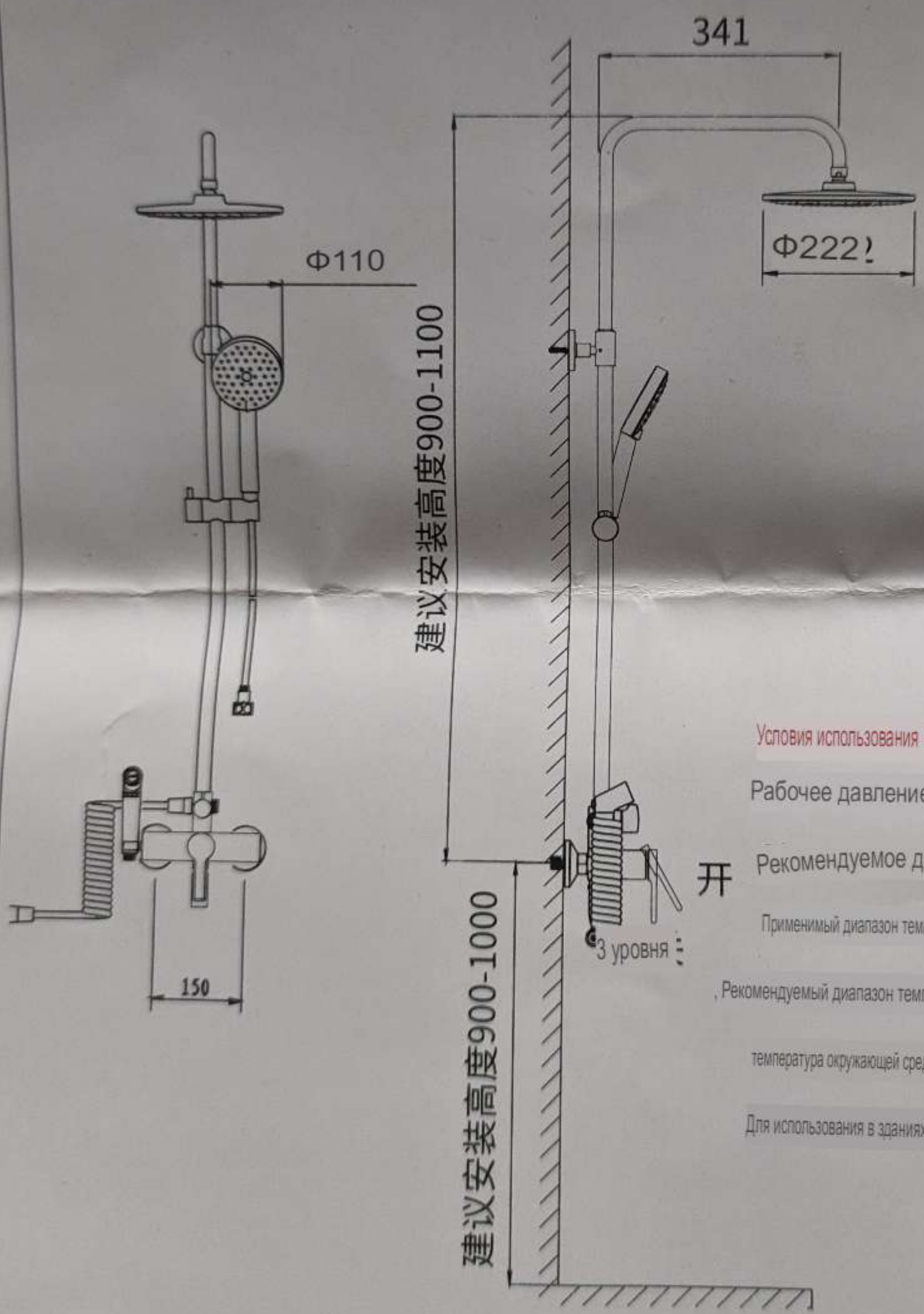
Схема размеров установки
